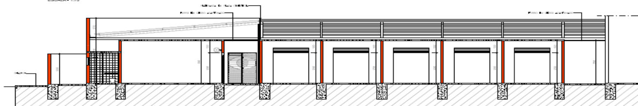
CORTE B.B ESCALA = 1/20
